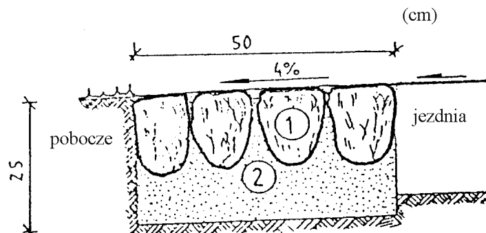
Rys. 1. Ob- ramowa- nie jezdni z brukow- ca 1. brukow- iec z kamie- nia łama- nego lub
