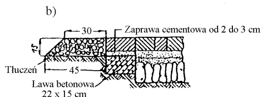
Rys. 5. Obramowanie jezdni z klinkieru ułożonego prostopadle do osi drogi
