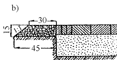
Rys. 4. Obramowanie jezdni z trze a) widok z góry b) przekrój poprzeczny
