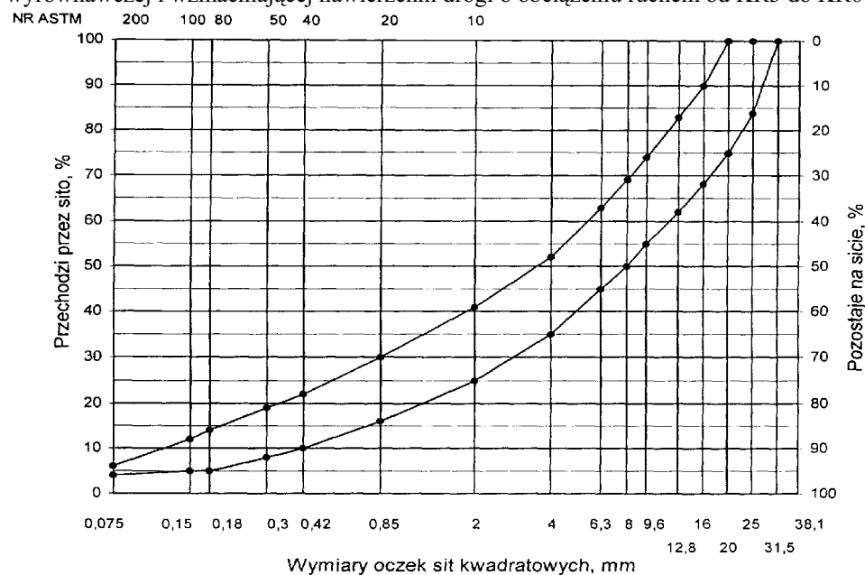
Rys. 12. Krzywe graniczne uziarnienia mieszanki mineralnej BA od 0 do 20 mm do warstwy wiążącej,
