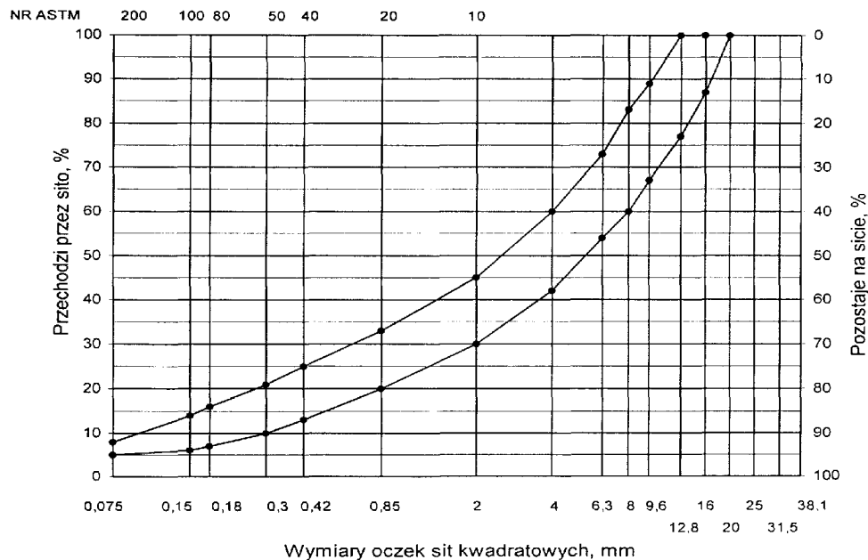
Rys. 12. Krzywe graniczne uziarnienia mieszanki mineralnej BA od 0 do 20 mm do warstwy wiążącej,
