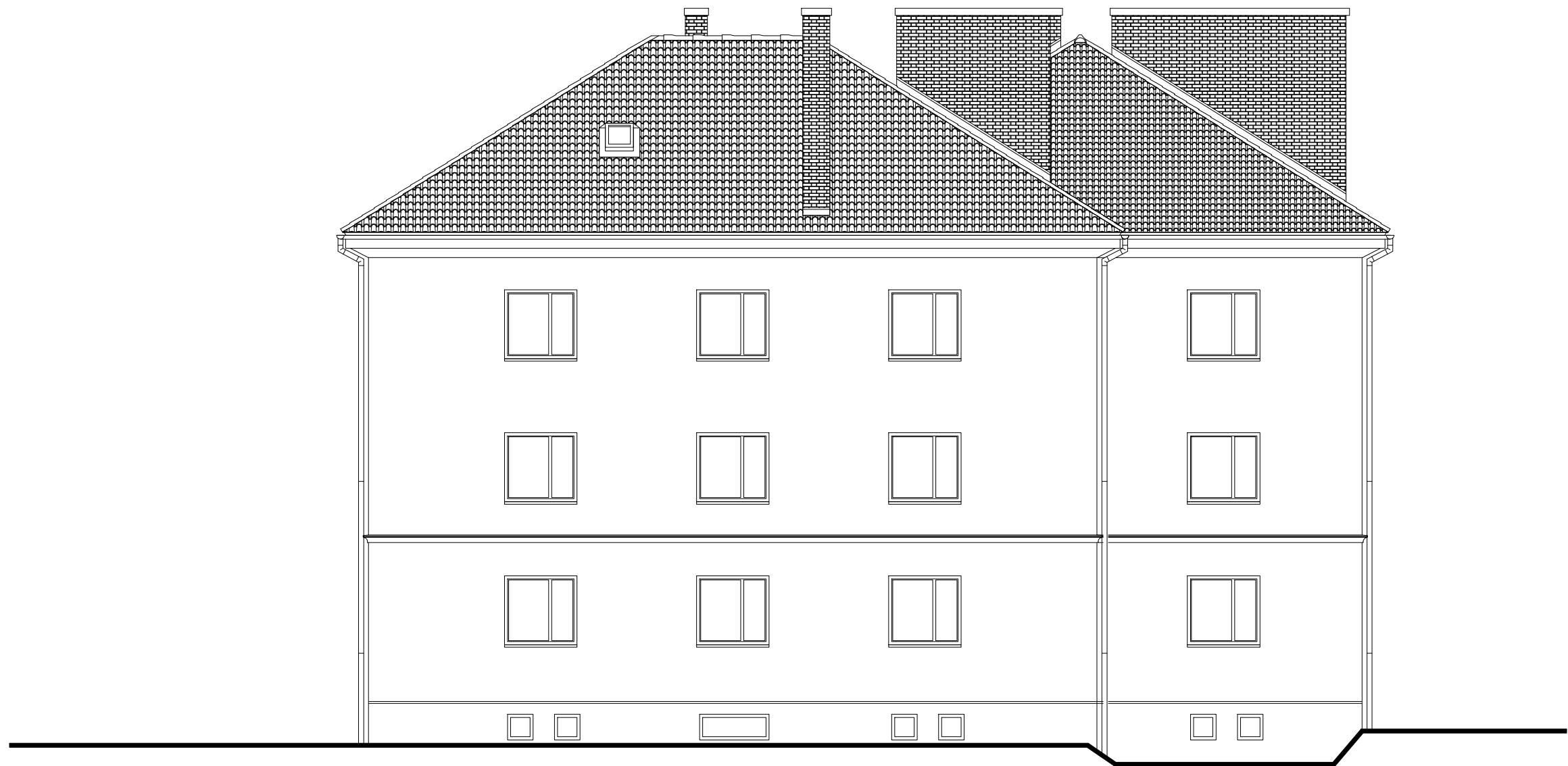
ELEWACJA ZACHODNIA
