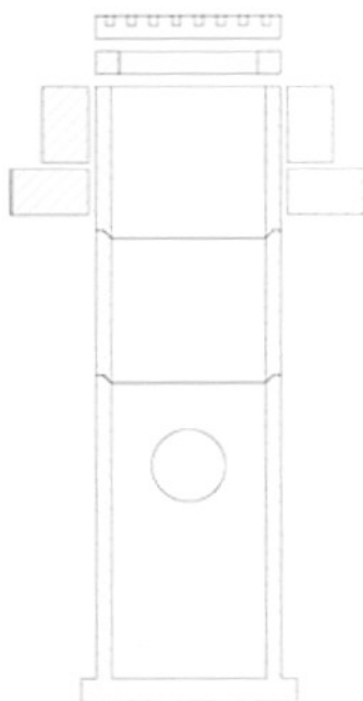
Rys. 2 Element prefabrykowany kompletu kraty ściekowej z osadnikiem 0,50m
